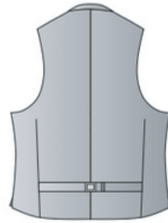
背中共生地 尾錠付きの場合薄生地のみ可 op 上下の+5%
